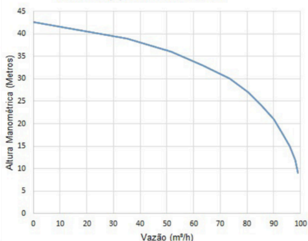
Curva do equipamento AQ-EL 44-100
